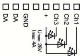
Anschlussplan 4A
