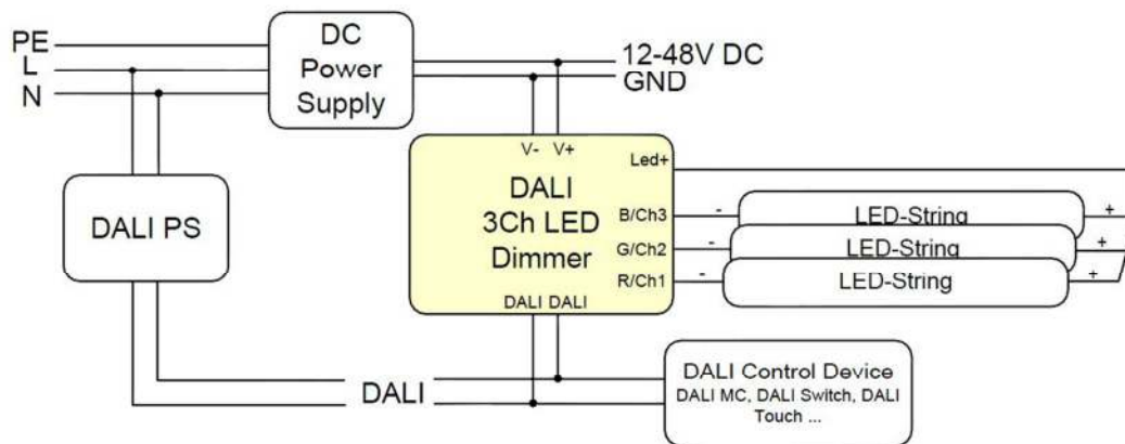
Prinzipschaltbild
