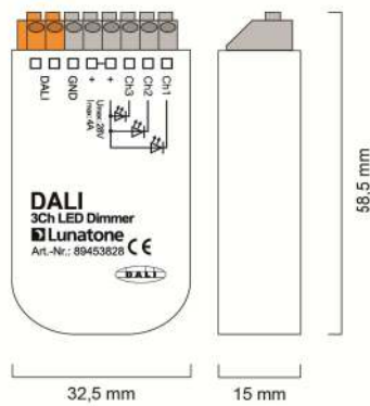
Geometrie 4A
